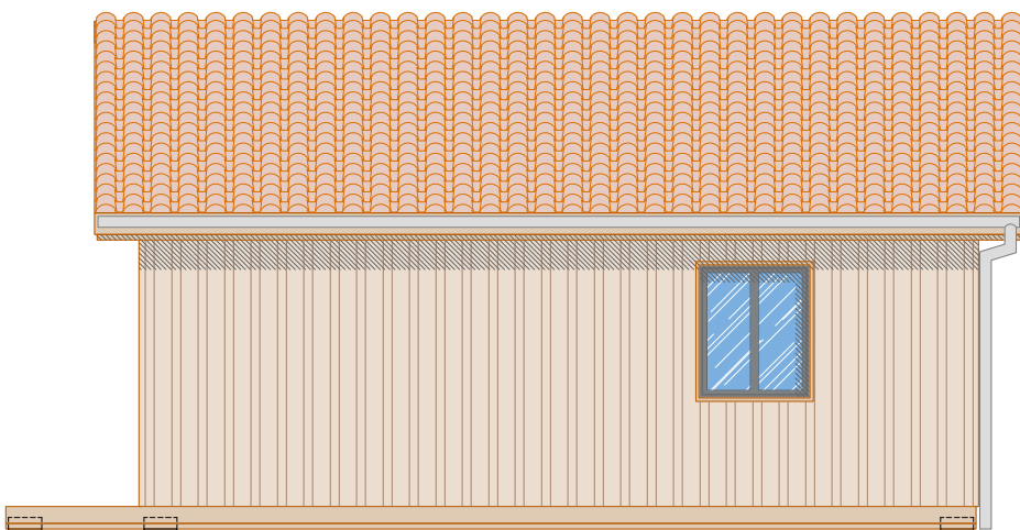
Façade OUEST
