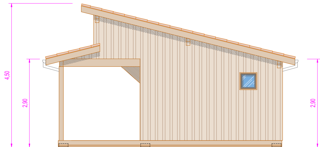
Façade NORD
