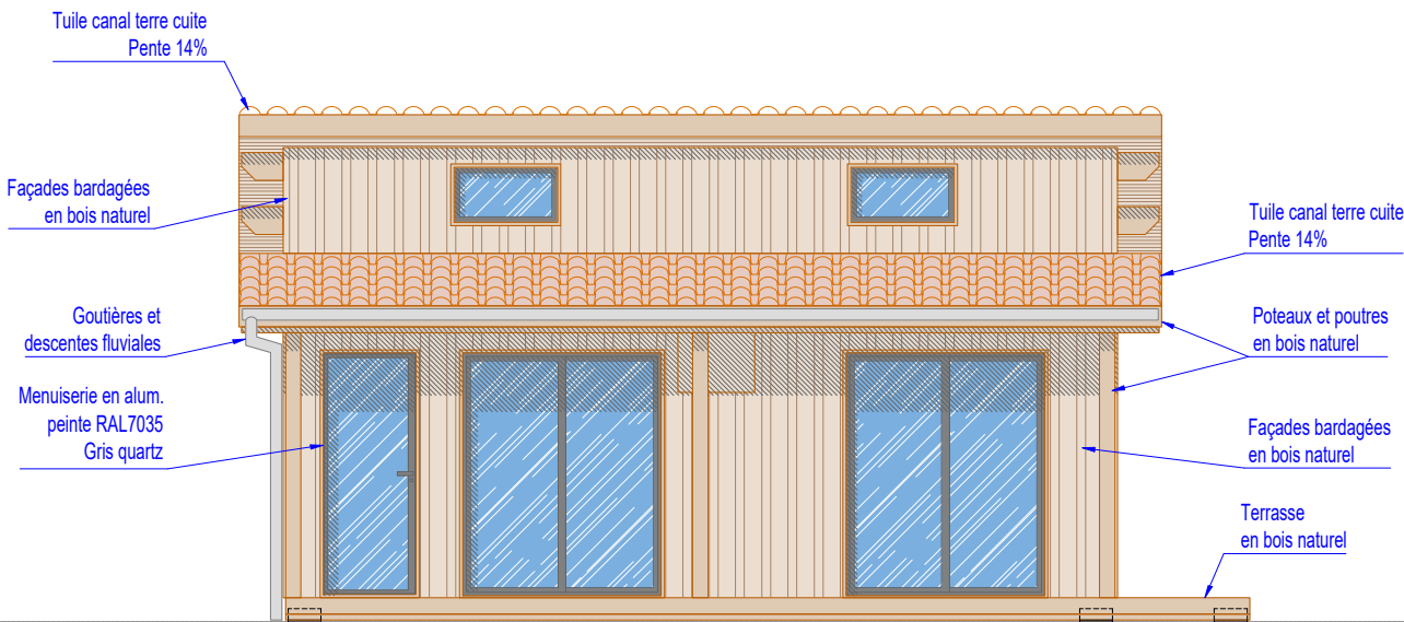
Façade EST
